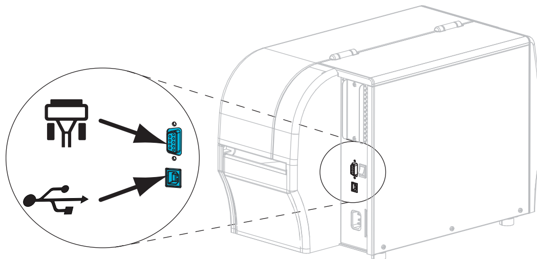
図 8・通信インターフェイス
