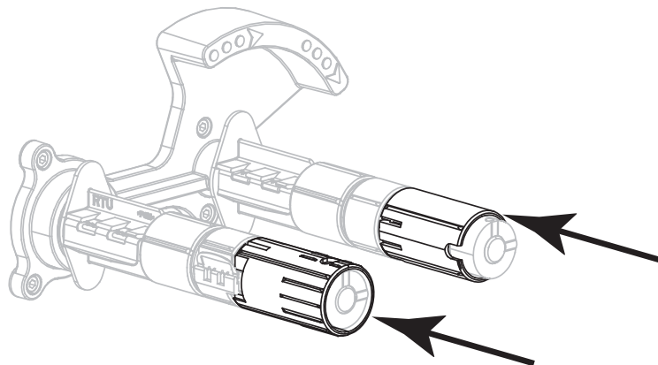
図 13・リボン・スピンドル — 低テンション設定（スピンドルのエンド・キャップを押し込んだ状態）
