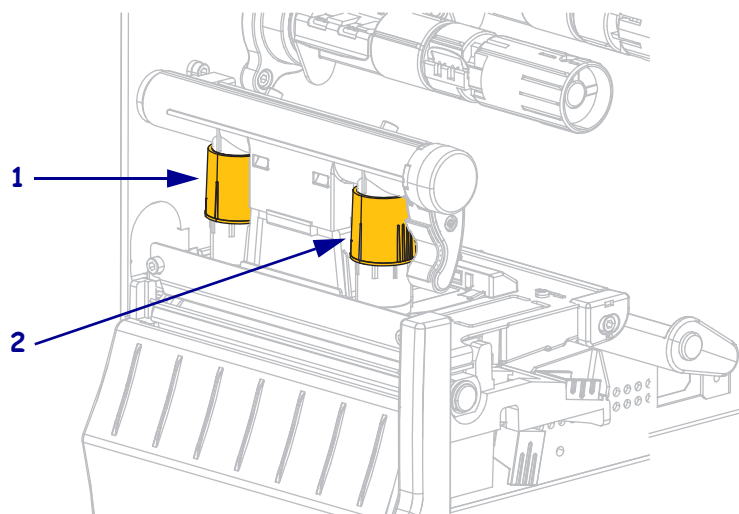
図 11・印字ヘッド圧力調整ダイヤル
