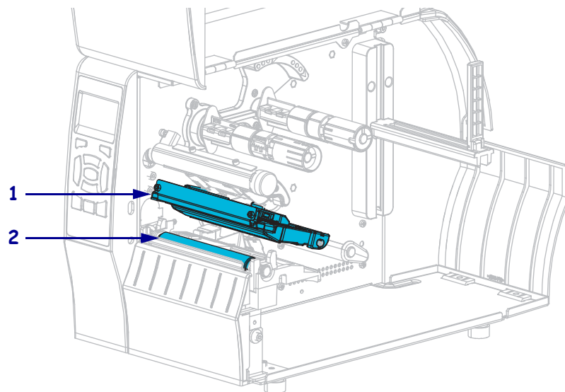
図 14・印刷ヘッドとプラテン・ローラーの場所
