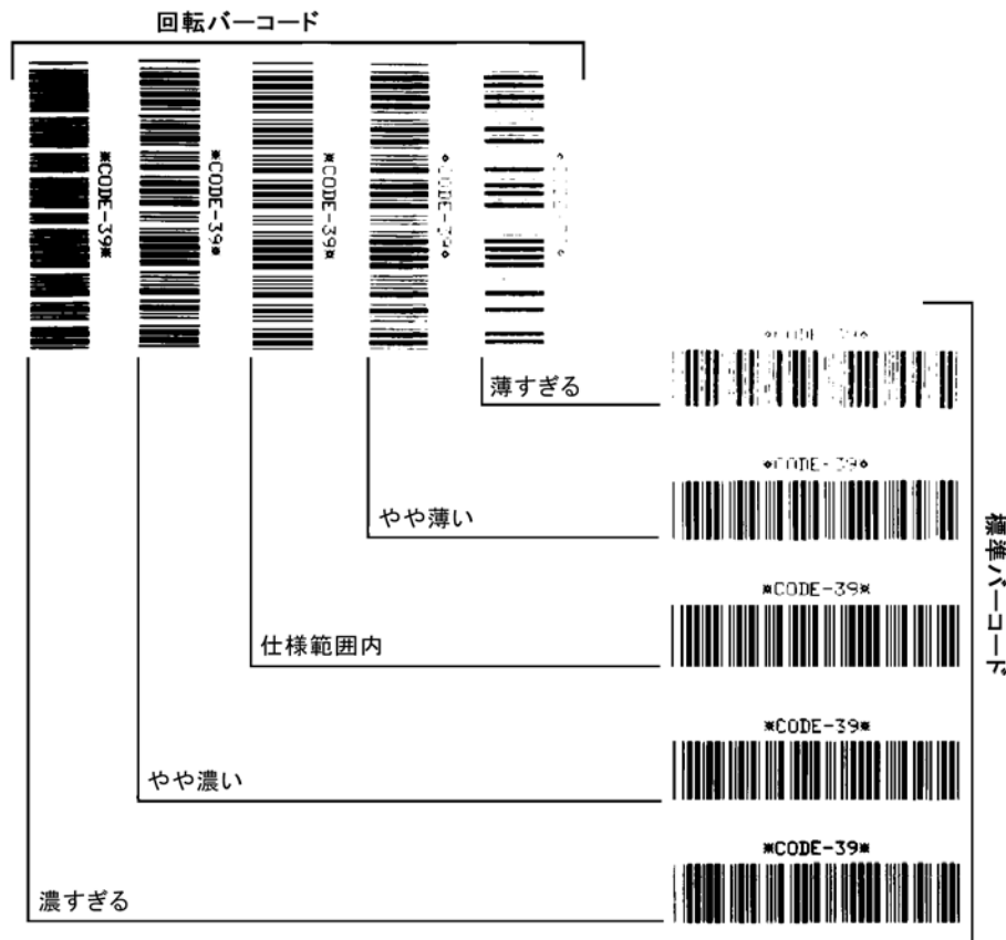
図 19・バーコードの濃度比較
